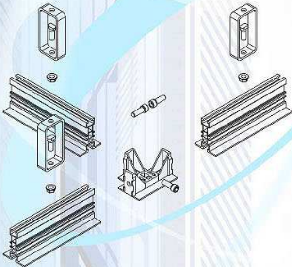
T 型接頭銜接分解表示圖 T BAR AND TYPE OF JUCTION
