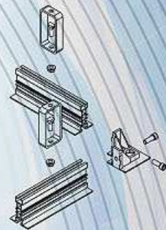
L 型接頭銜接分解表示圖 T BAR AND TYPE OF JUCTION
